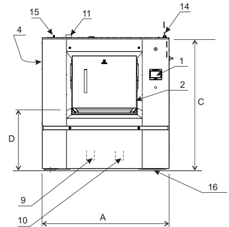
Vooraanzicht
